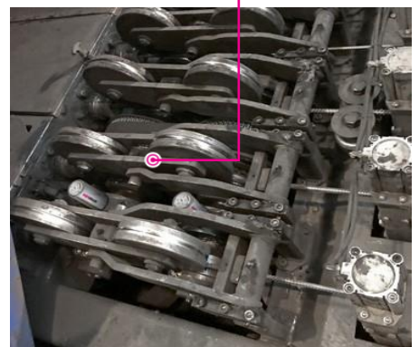
simalube 125ml 자동주입기가 6개월로 설정되어 절단 기계의 공급 장치에 연결되어 있습니다.
